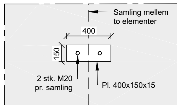
Detail A: Principforslag samling ml. elementer, 1:20
