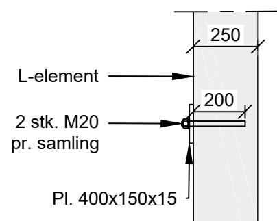
Detail B: Principforslag samling ml. elementer, 1:20
